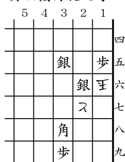
例題 4 安北協力詰 5 手
